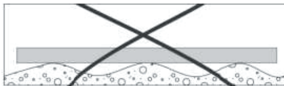
Рисунок 1. Укладка на грунт, в т.ч. и на песчано-гравийную подушку, НЕДОПУСТИМА!
